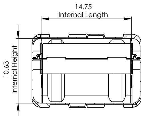
SECTION B-B SCALE 1 : 9
