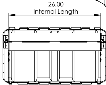
SECTION B-B SCALE 1 : 14
