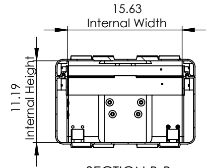
SECTION B-B SCALE 1 : 13
