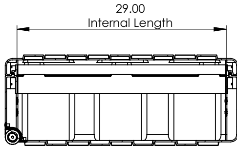
SECTION A-A SCALE 1 : 13
