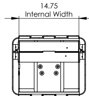
SECTION B-B SCALE 1 : 14
