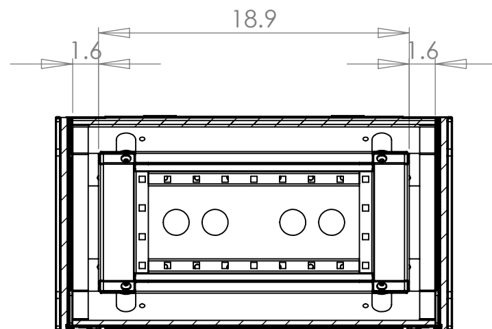
SECTION A-A SCALE 1 : 8
